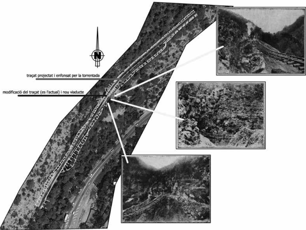
Enfonsament que es va produir a les vies de el ferrocarril de Sóller a causa d'una torrentada el 05-10-1919
